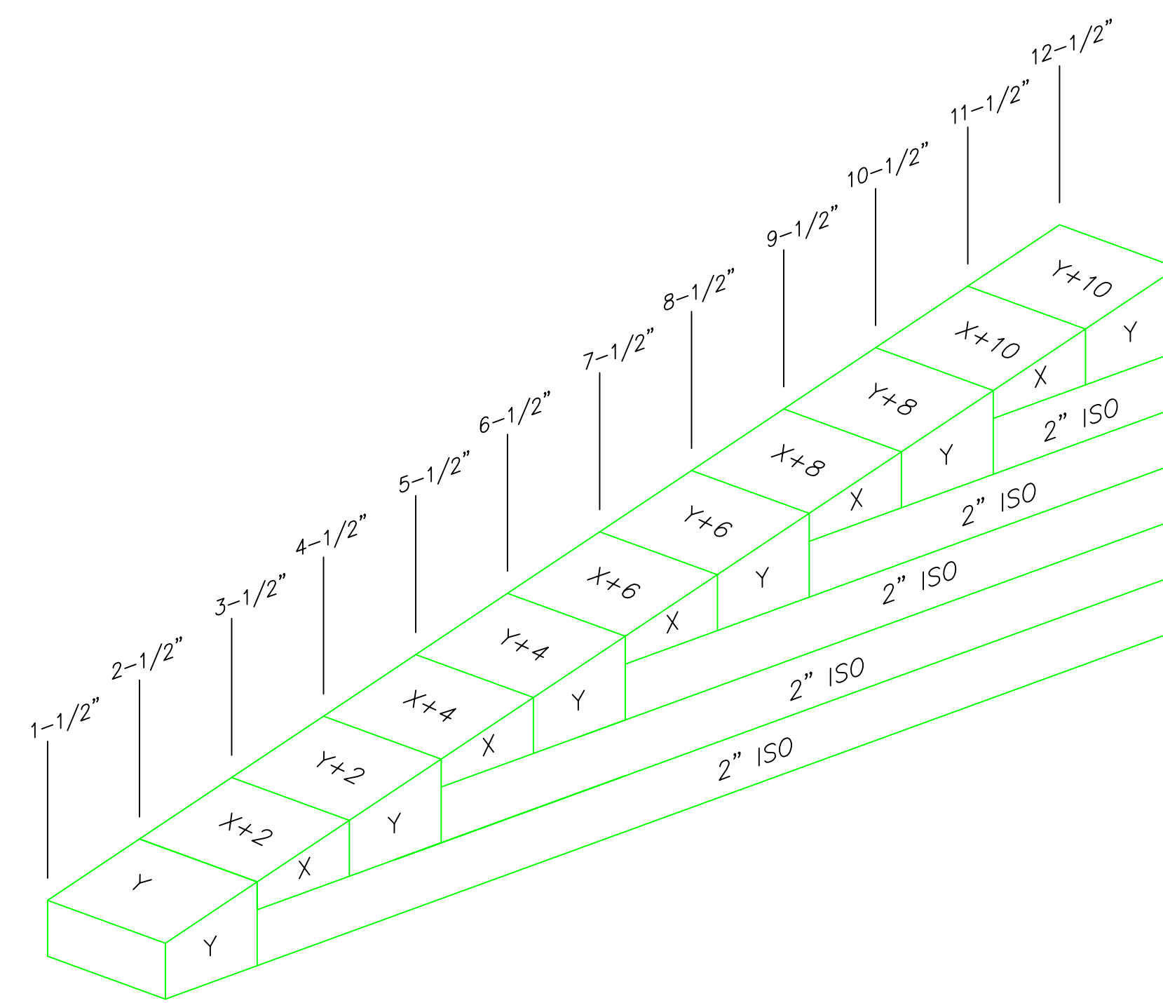
1/4" PER FT TAPERED ISO SCALE: NTS
