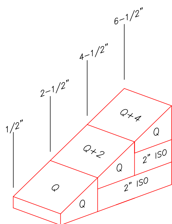
1/2" PER FT TAPERED ISO SCALE: NTS
